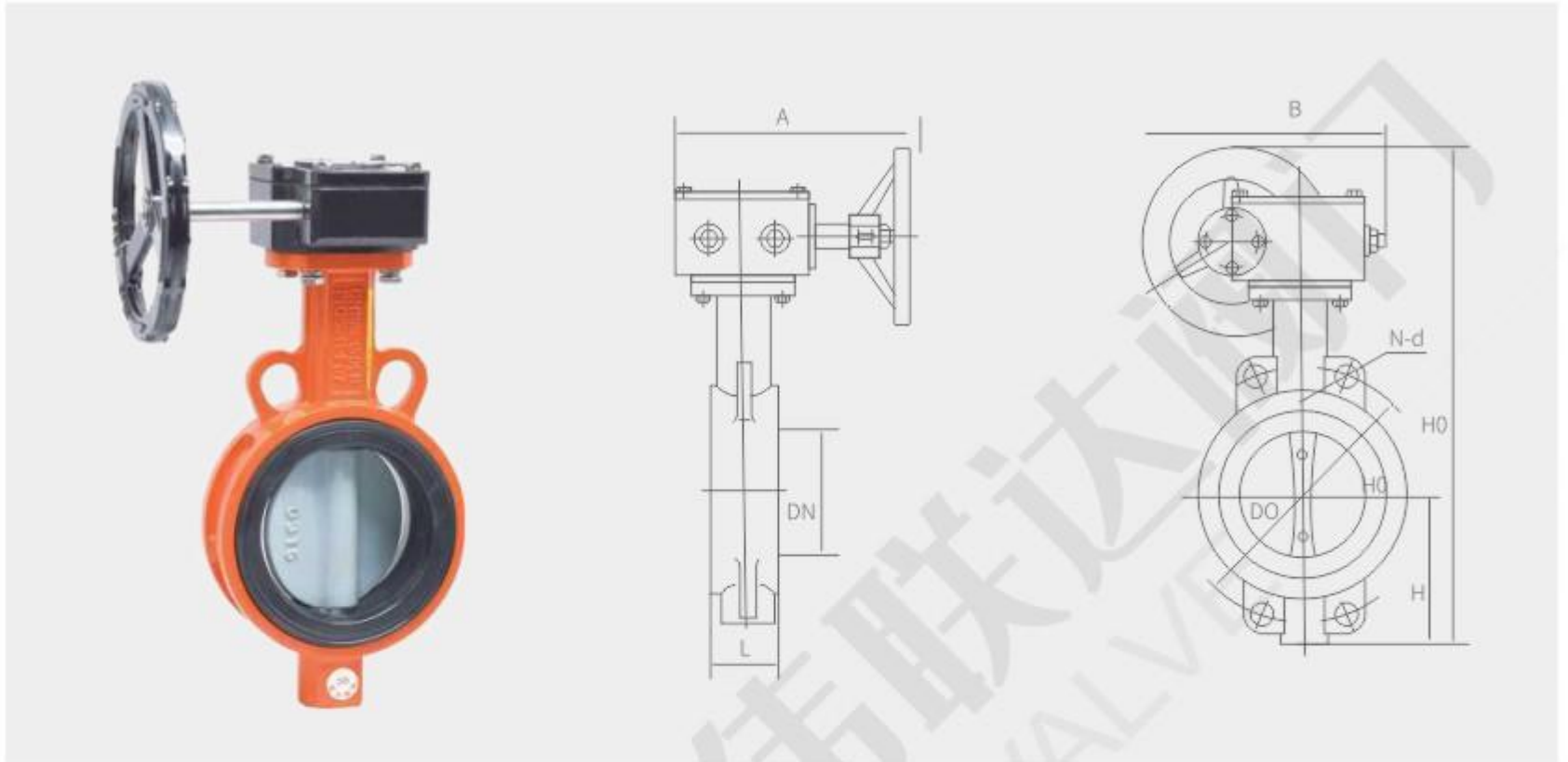
D371X- 6 / 10 对夹蜗轮软密封蝶阀主要外形连接尺寸
