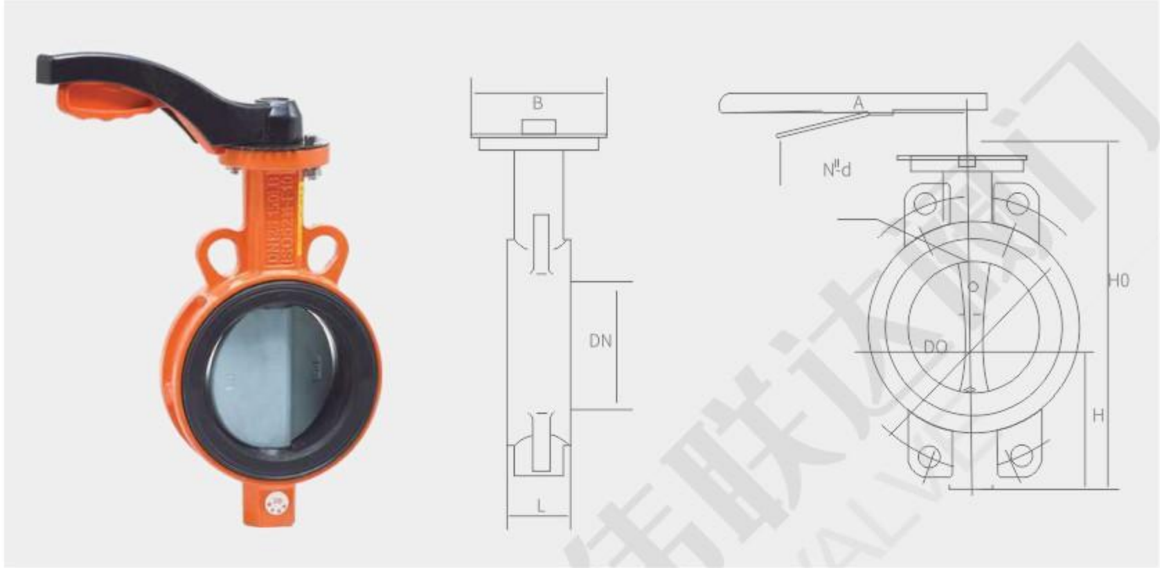
D71X- 6 / 10 对夹软密封蝶阀主要外形连接尺寸
