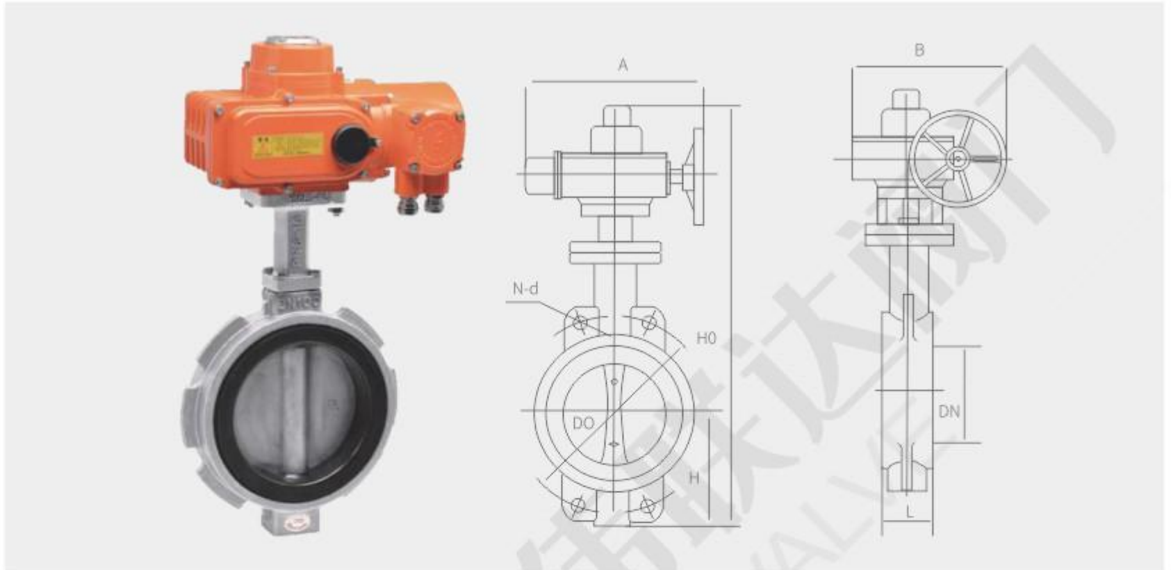
D971X- 6 / 10 对夹电动软密封蝶阀主要外形连接尺寸 16
