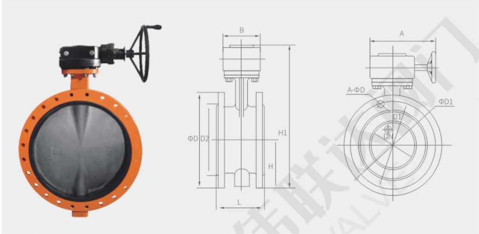
D341X (FBGX) 蜗轮传动软密封蝶阀主要外形连接尺寸
