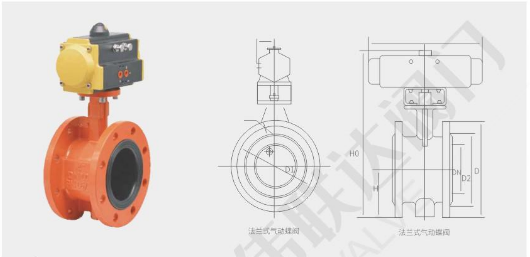
D641X - 6 / 10 / 16 气动软密封蝶阀主要外形连接尺寸
