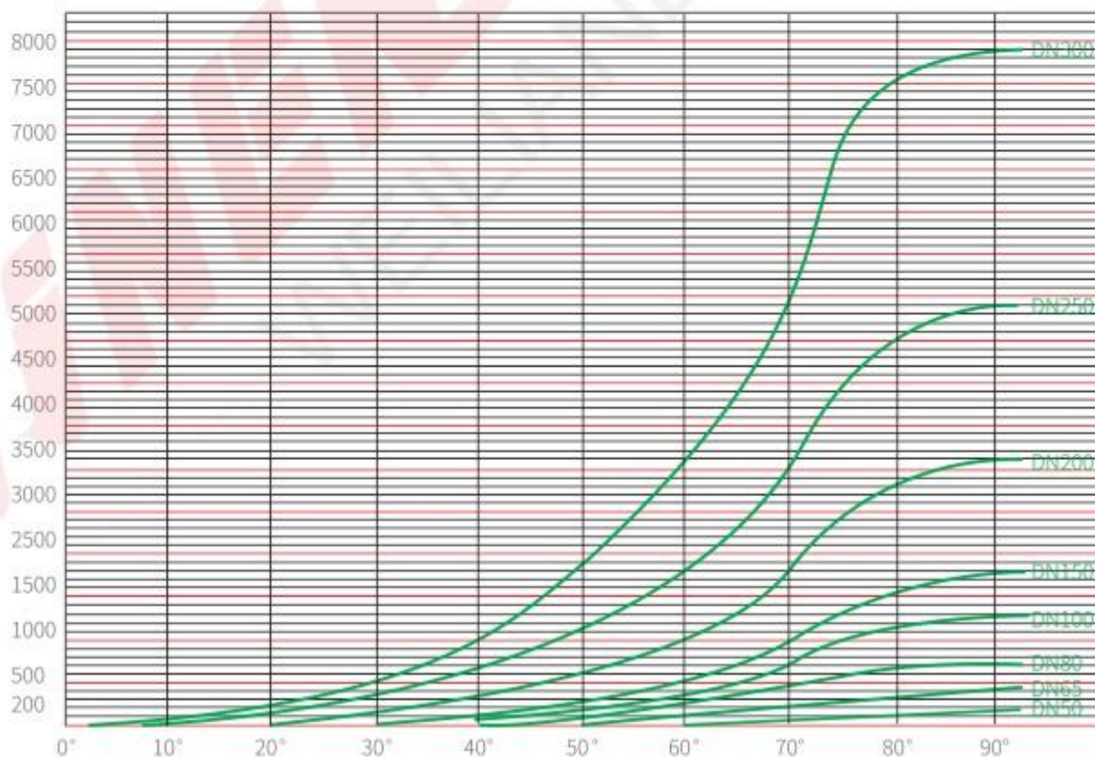
曲线流量图 Curve flow chart
