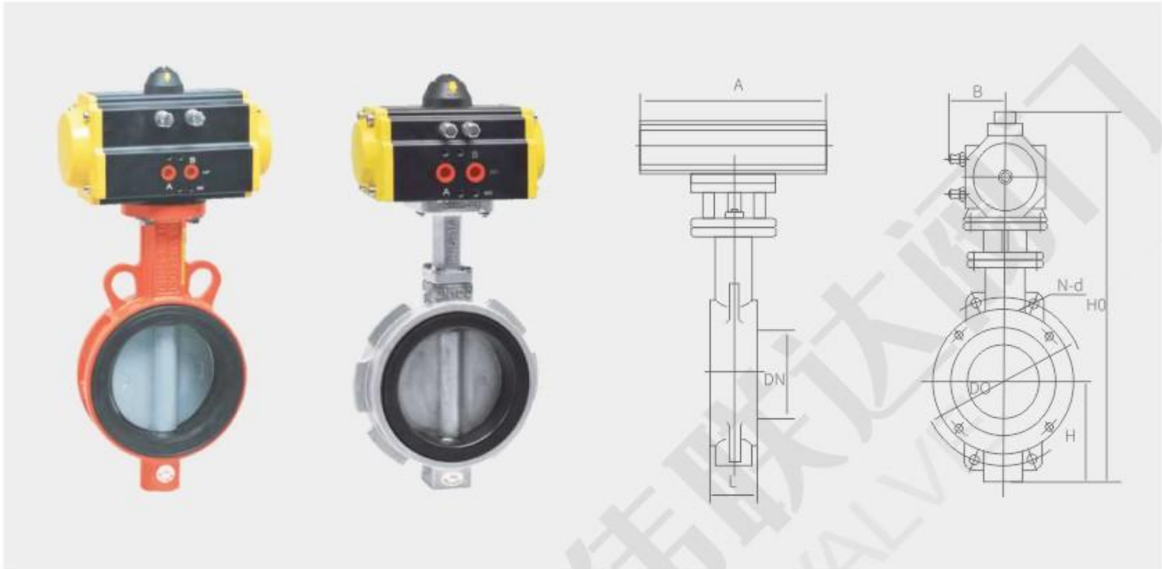
D671X- 6 / 10 / 16 对夹气动软密封蝶阀主要外形连接尺寸
