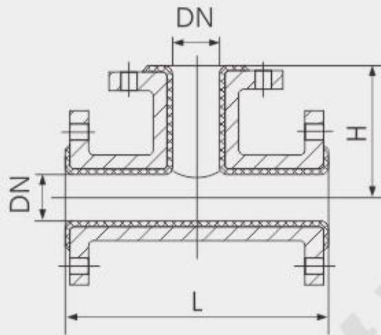
等径三通管
