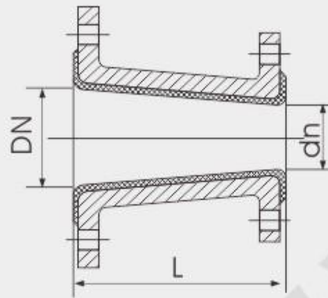
同心异径管
