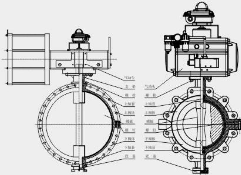
图一单作用气动衬氟蝶阀
